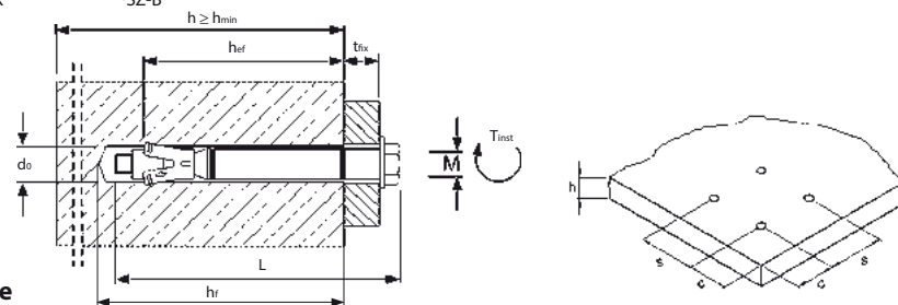
Maße Senkkopf für SZ-SK A4 [mm]
